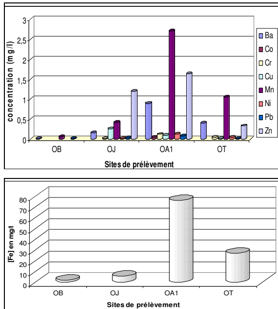
Figure 7 : Évolution des métaux lourds en (mg/l).
