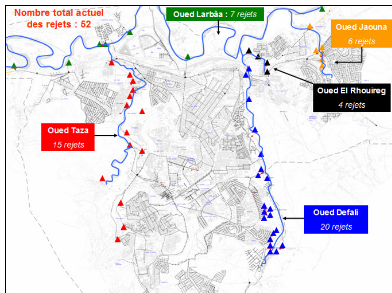
Figure 1 : Le réseau d'assainissement de la ville avec emplacement des rejets (RADEETA)
