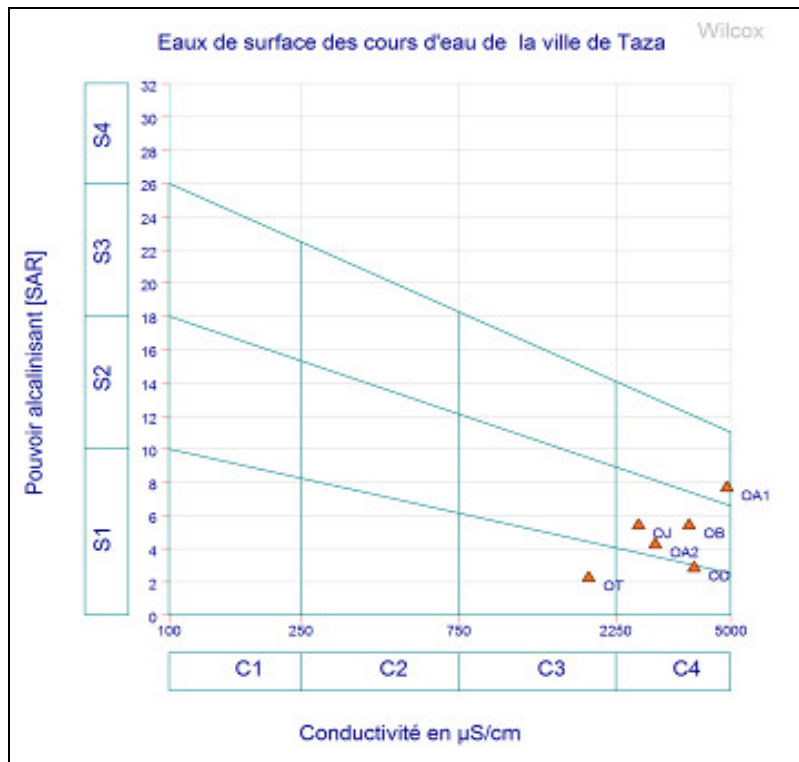
Figure 9 : Diagramme de WILCOX des différents points d'eau
