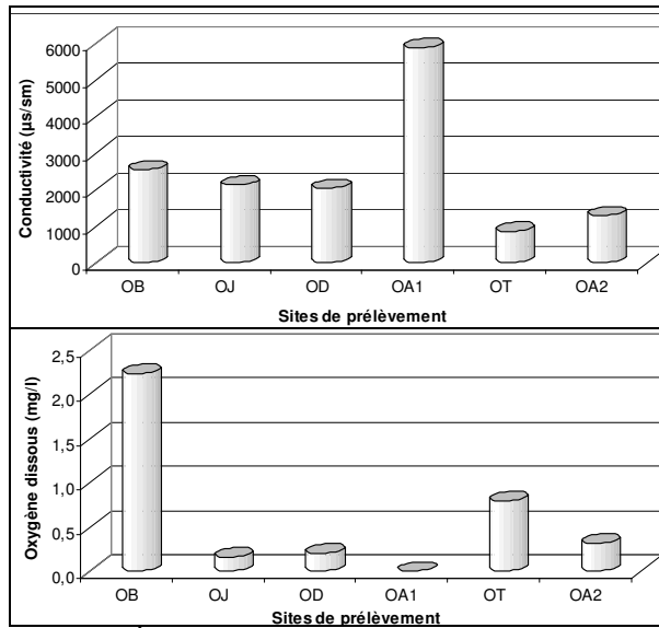
Figure 3 : Évolution de la conductivité et de l'O 2 dissous.
