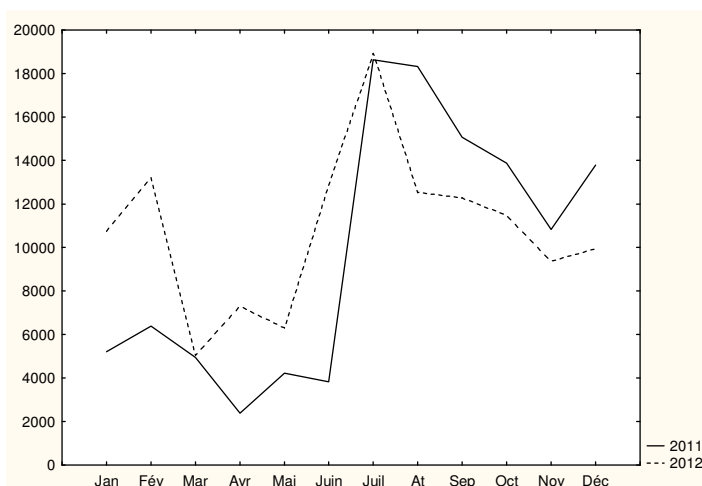
Figure 2 : Graphique présentant les variations mensuelles du peuplement d'Oiseau.
