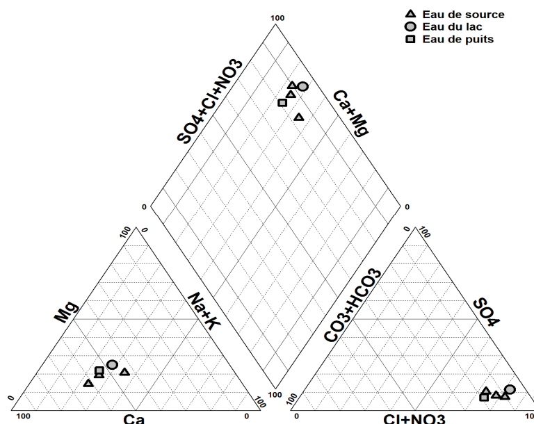
Figure 5. Classification hydrochimique des eaux de Mangouin-Yrongouin
