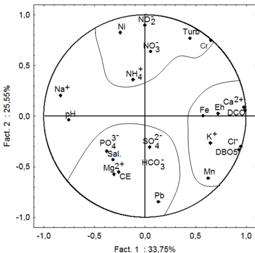
Figure 6. Analyse dans le plan factoriel F1-F2
