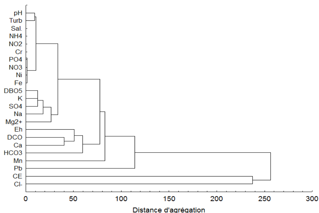
Figure 7. Dendrogramme des paramètres physico-chimiques des eaux de Mangouin-Yrongouin
