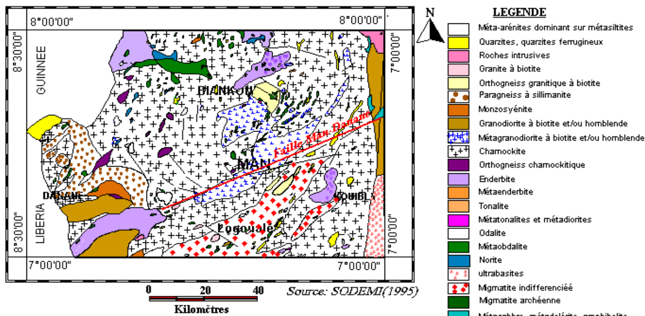
Figure 2 : Carte géologique de la région de Man-Biankouman (Saley, 2003)
